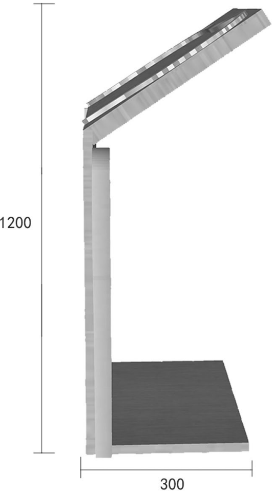
【侧视图】
