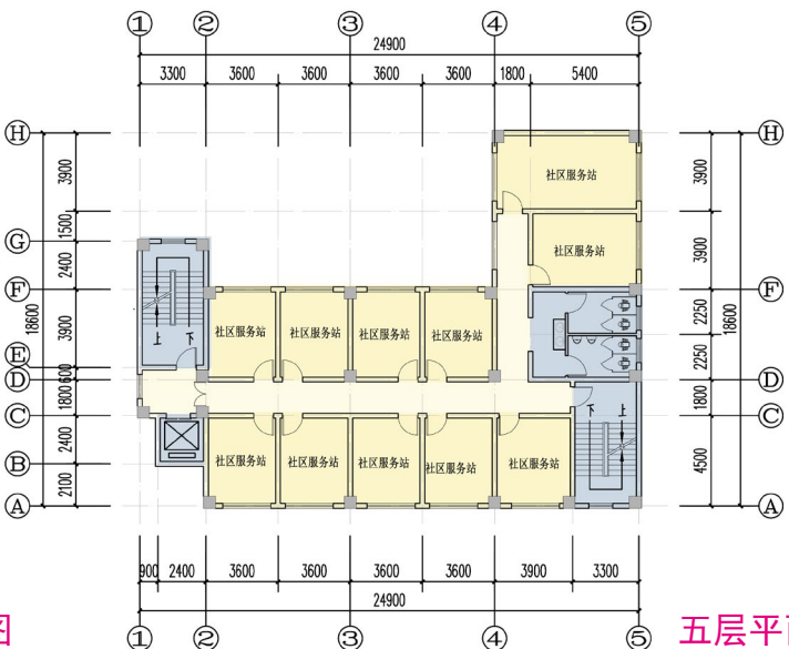
四层平面图
