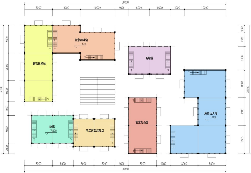
三层平面图
