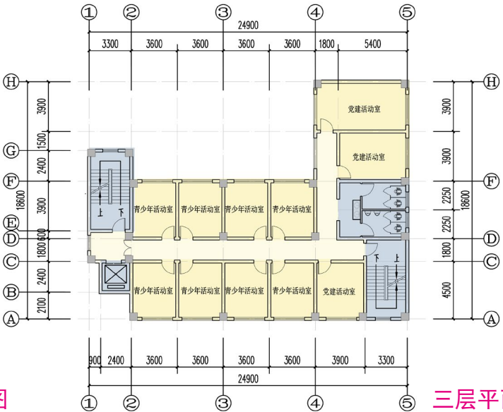
二层平面图
