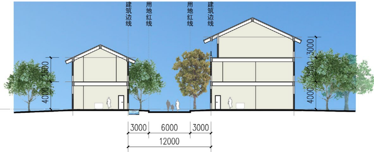
二级商业街 街道宽度 12m
