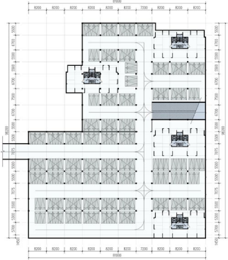
5# 停车库平面图 本层建筑面积 6800m 2 机动车停车位 250 个
