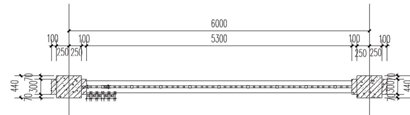
围墙平面图
