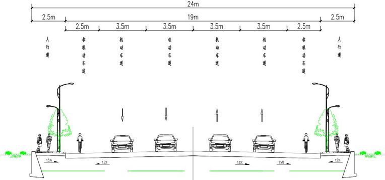
城市次干道标准横断面图
