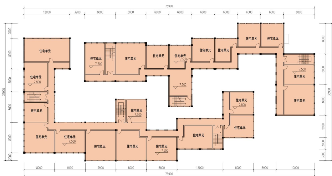
三层平面图
