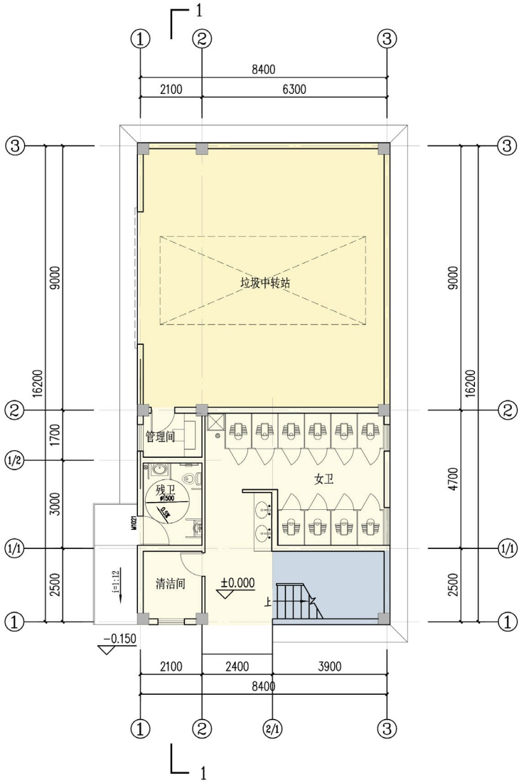
一层平面图
