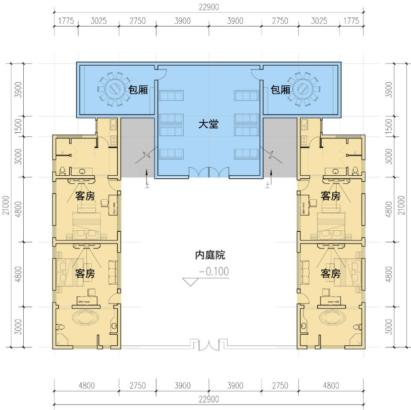
一层平面图
