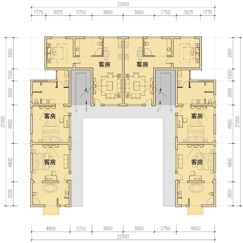
二层平面图
