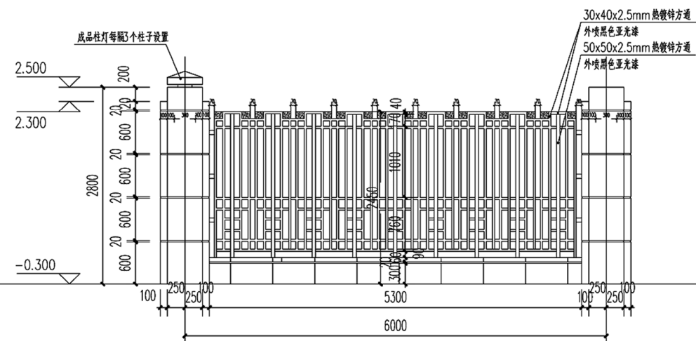
围墙立面图
