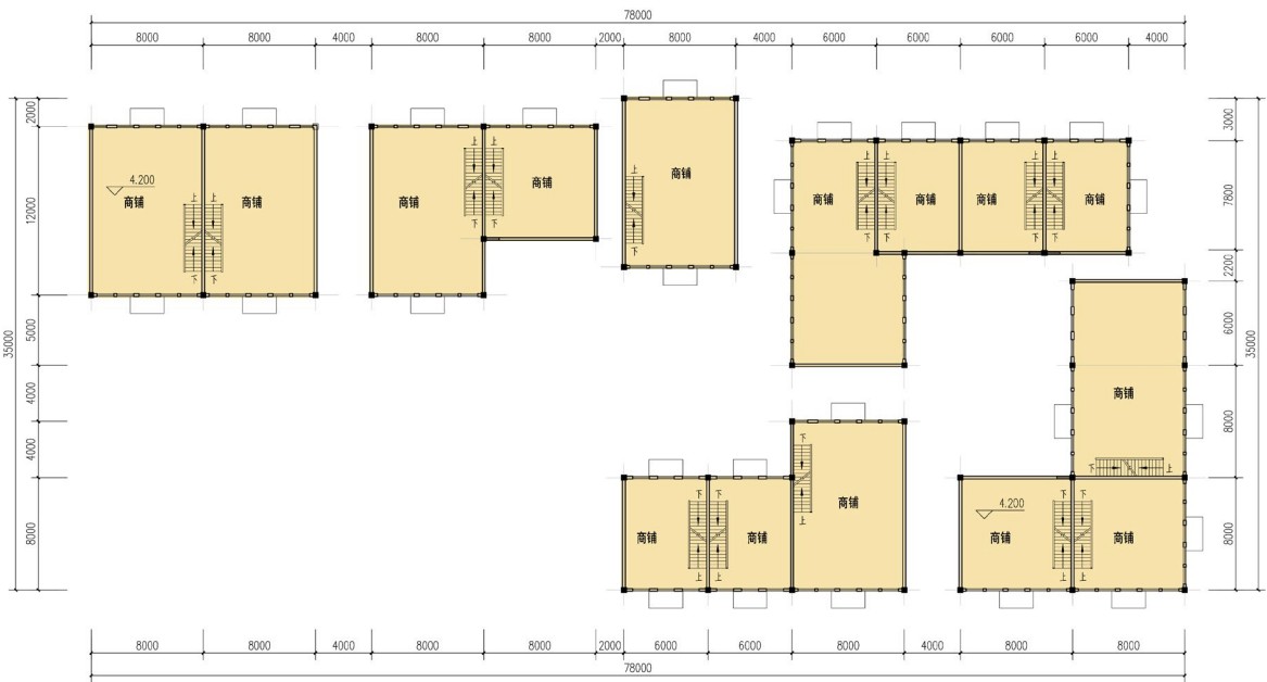
二层平面图
