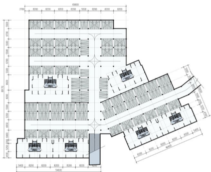
6# 停车库平面图 本层建筑面积 7380m 2 机动车停车位 240 个
