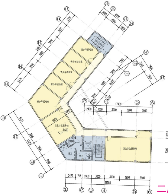
一层平面图
