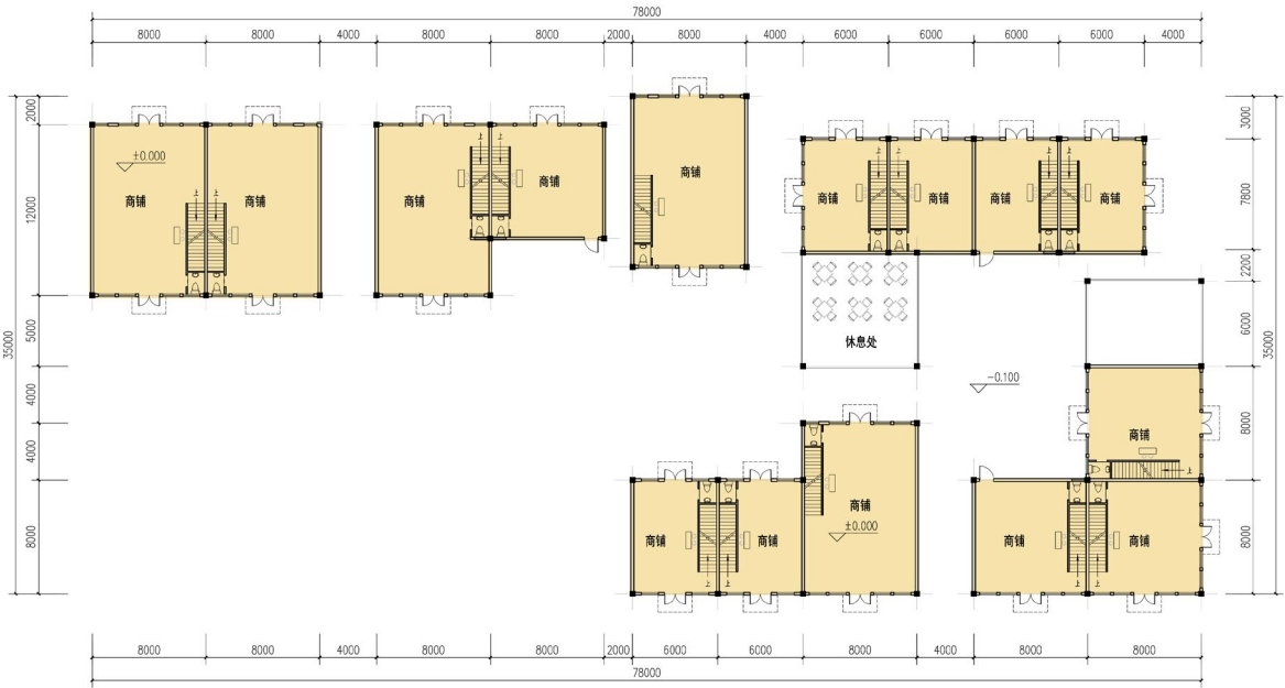
一层平面图
