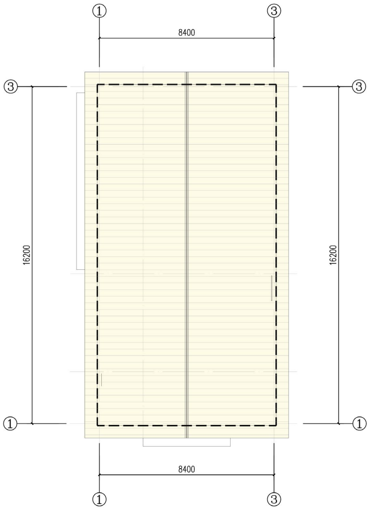
屋顶层平面图
