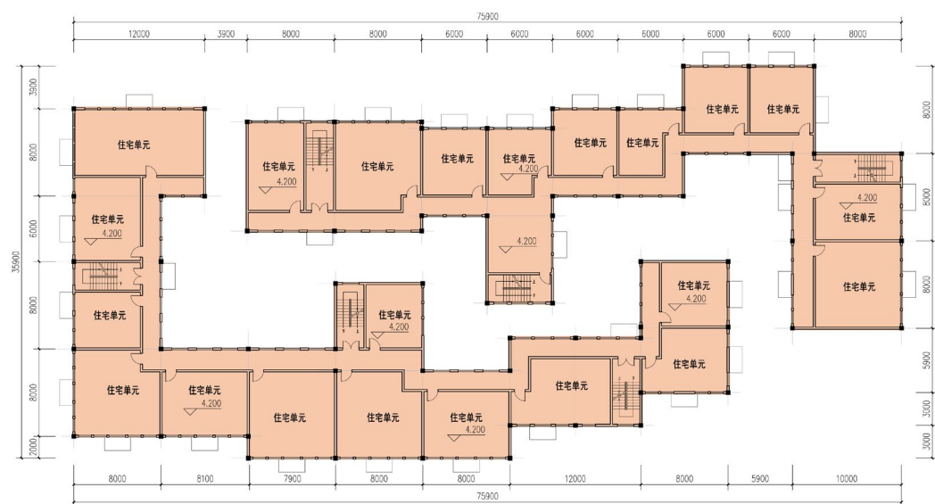
二层平面图
