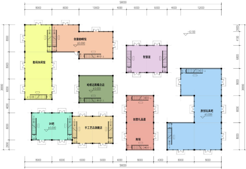
一层平面图
