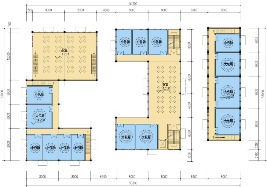
二层平面图
