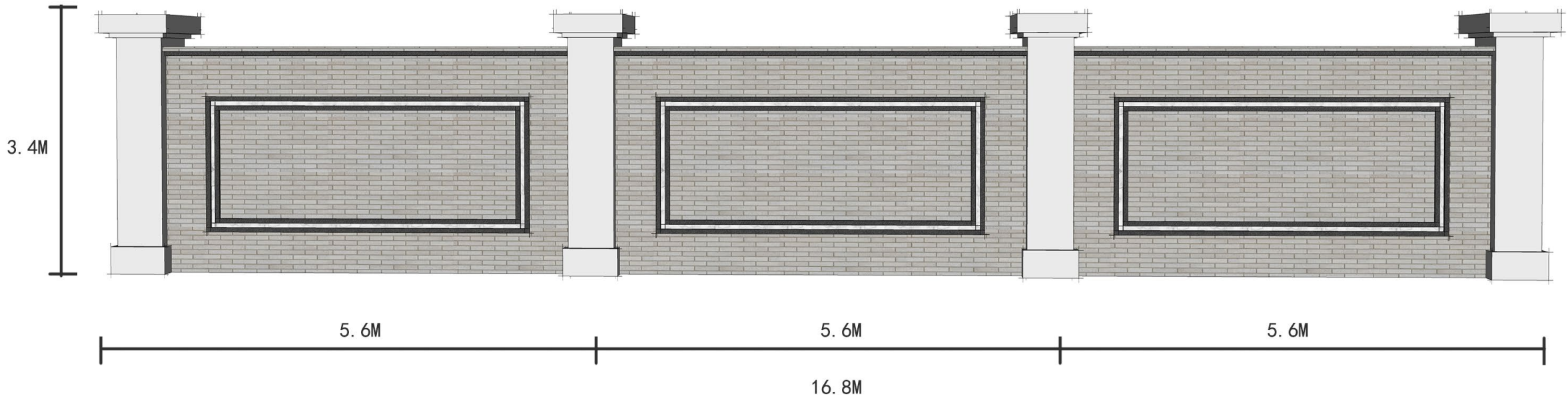
风貌协调过渡区围墙形式一
