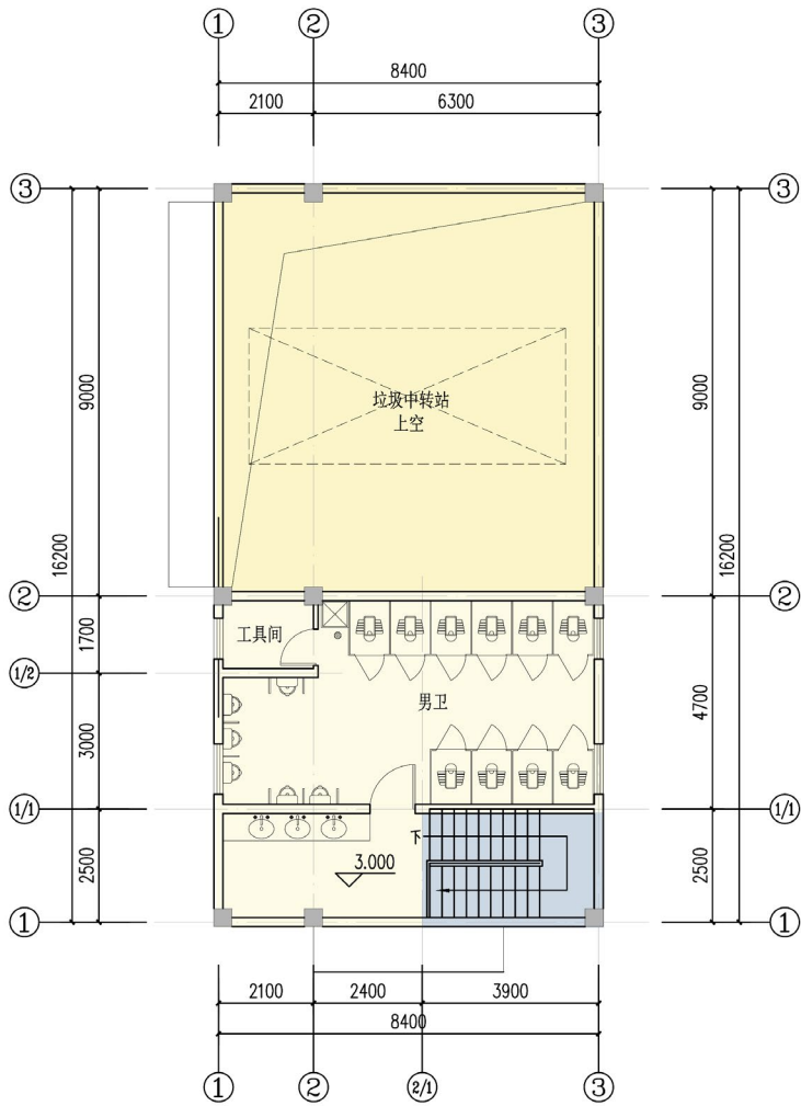
二层平面图
