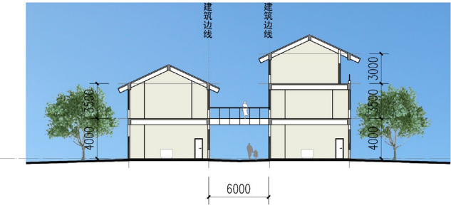
三级商业街 街道宽度 6m
