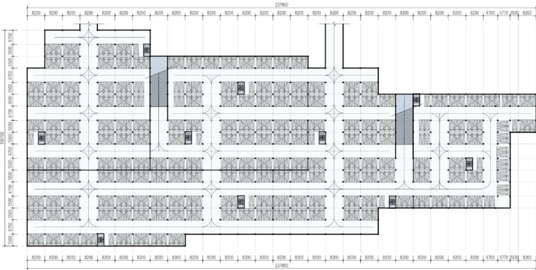
4# 停车库平面图 本层建筑面积 18000m 2 机动车停车位 890 个
