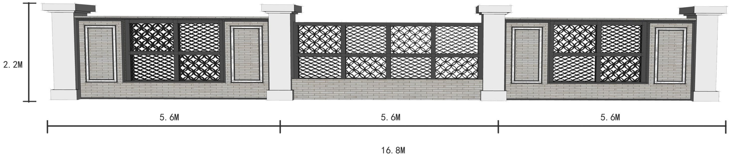
风貌协调过渡区围墙形式二
