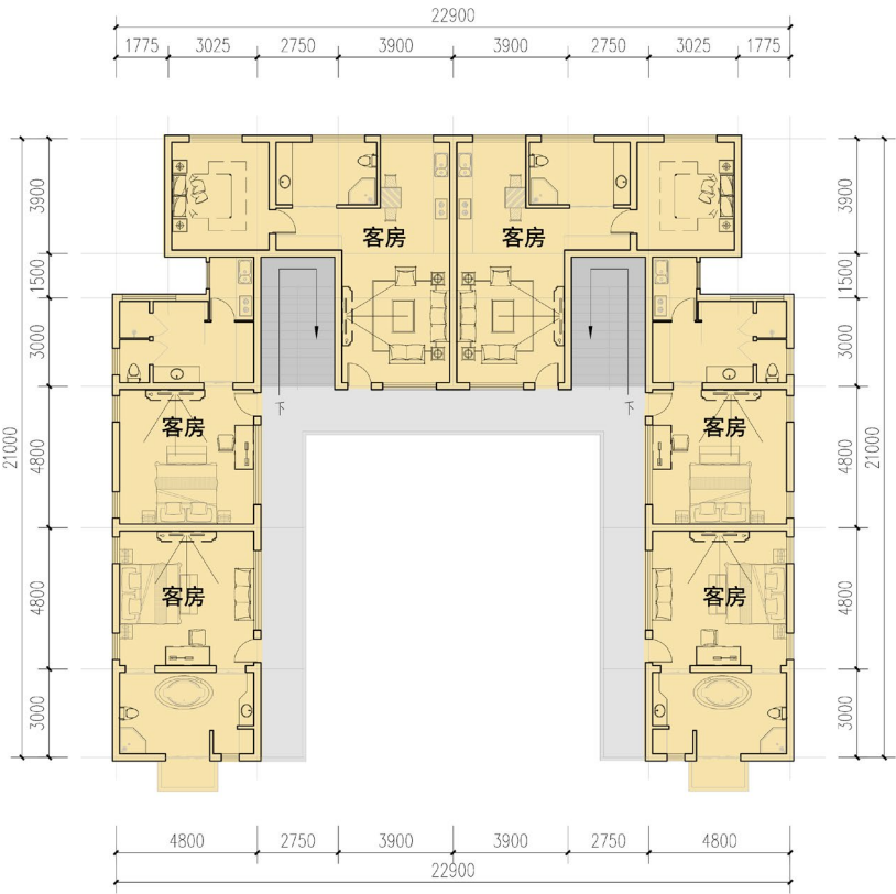
三层平面图
