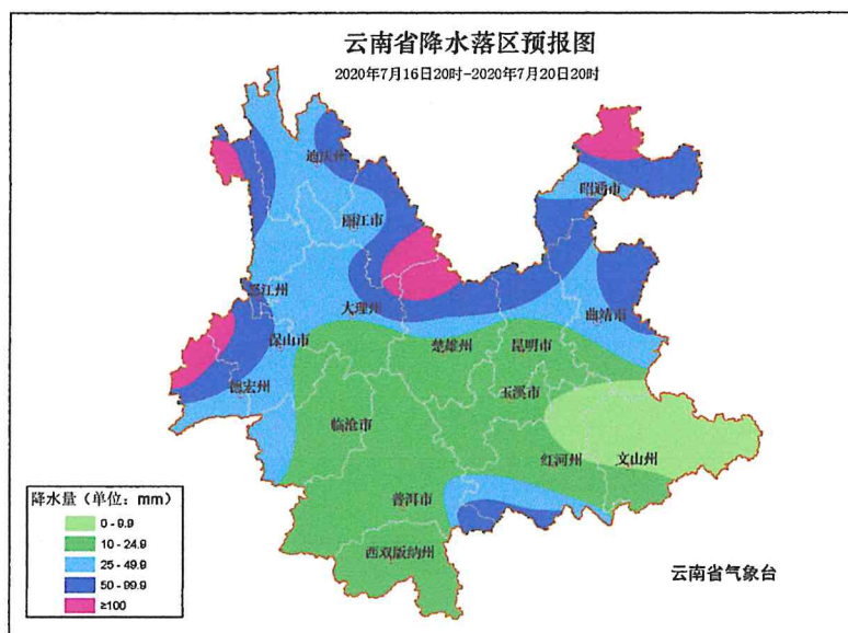
7月16日20时至7月20日20时降水量预报图
